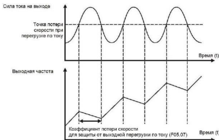
Рис. 6.11 — График работы защиты от перегрузки по току
