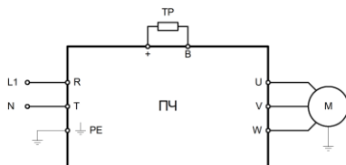
Рис. 3.2.3 — Подключение силовых клемм для моделей LCI-GY/PY-2B(S)
