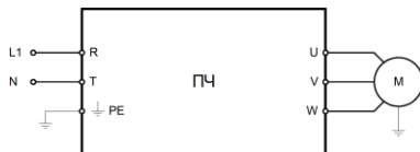
Рис. 3.2.4 — Подключение силовых клемм для моделей LCI-GY/PY-3
