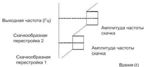
Рис. 6.18 — Скачкообразная перестройка частоты
