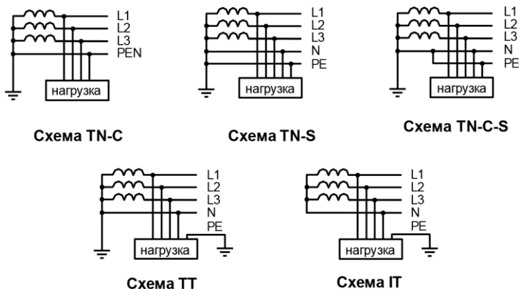
Рис. 3.6 – Типы систем заземления.
