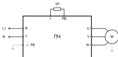
Рис. 3.2.2 — Подключение силовых клемм для моделей LCI-GY/PY-2(B)
