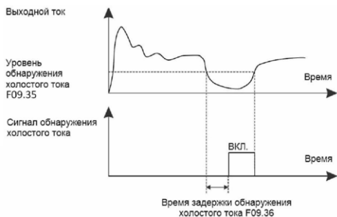
Рис. 6.21 — Обнаружение холостого тока
