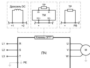
Рис. 3.2.6 — Подключение силовых клемм для моделей LCI-GY/PY-4(B)
