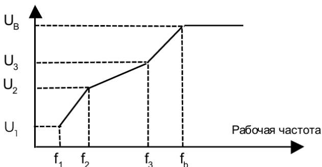
Рис. 6.7 – Ломаная характеристика U/f
