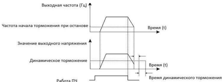
Рис. 6.4 - Процесс торможения постоянным током
