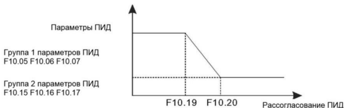
Рис. 6.25 — Рассогласование ПИД
