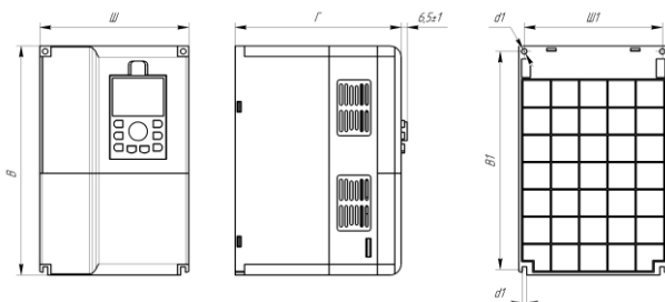
Рис. 2.5 — Габаритные и установочные размеры устройств серии LCI в пластмассовом корпусе
