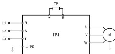
Рис. 3.2.5 — Подключение силовых клемм для моделей LCI-GY/PY-4B(S)
