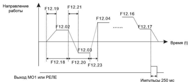
Рис. 6.28 — Направление работы ПЧ
