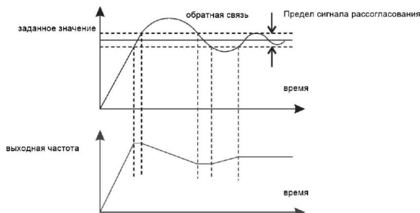
Рис. 6.24 — Отклонение ПИД-управления
