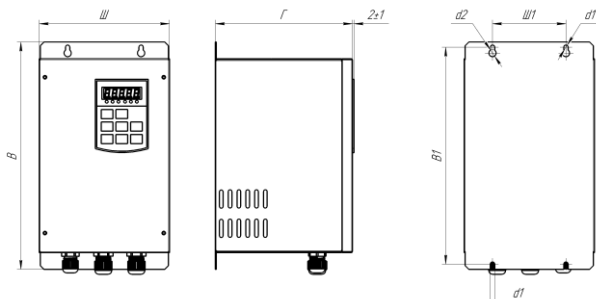
Рис. 2.8 — Габаритные и установочные размеры устройств серии LCI в корпусе IP54/IP55
