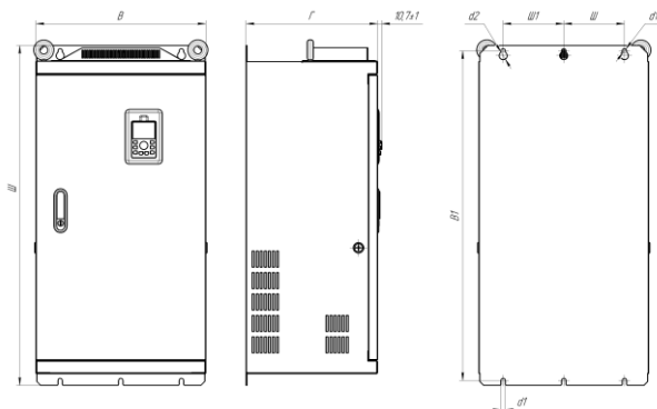
Рис. 2.6 — Габаритные и установочные размеры устройств серии LCI в металлическом корпусе
