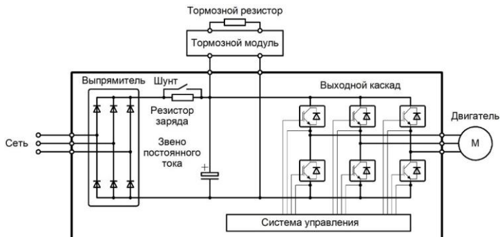
Рис. 2.2 – Принципиальная электрическая схема моделей свыше 30 кВт (включительно)
