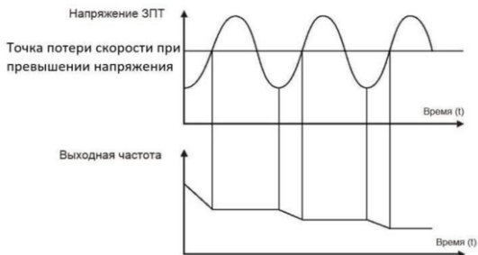
Рис. 6.10 — График работы защиты от перенапряжения
