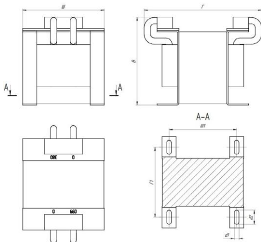
Рис.2.7 — Габаритные и установочные размеры разделительного трансформатора для моделей LCI-GY/PY-6
