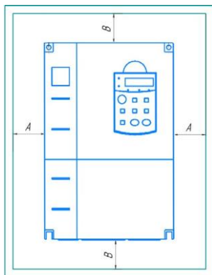
Рис. 3.1 — Требуемые расстояния при монтаже
