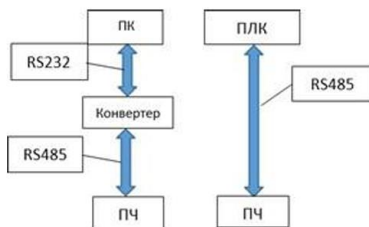
Рис. 7.1 Сетевой режим Master/Slave
