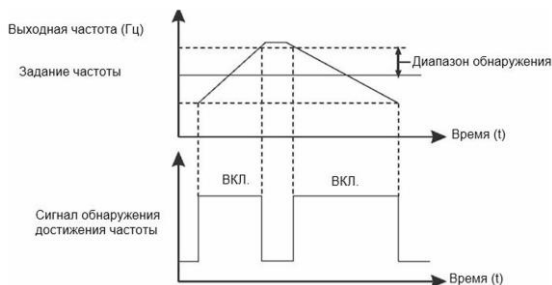
Рис. 6.17 — Диапазон достижения максимальной частоты
