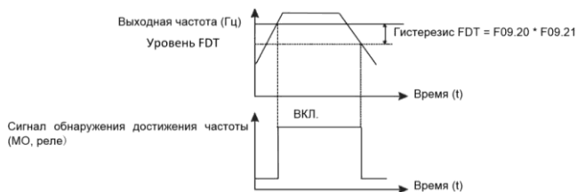
Рис. 6.16 — Значения обнаружения выходной частоты
