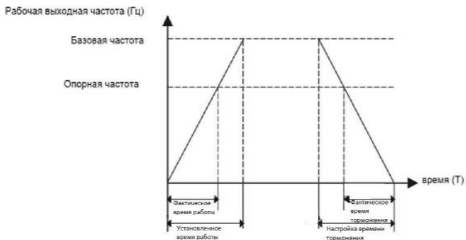
Рис. 6.1 - Время разгона/торможения
