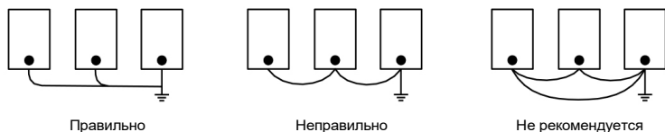
Рис. 3.5 — Схематичное изображение образования петли с заземляющим проводом
