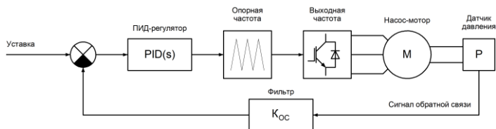
Рис. 6.23 — Схема ПИД-регулирования
