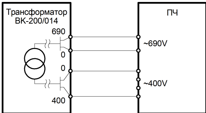
Рис. 3.2.8 – Схема подключения разделительного трансформатора для моделей LCI-GY/PY-6
