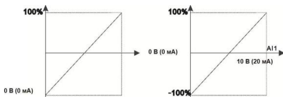
Рис. 6.12 — Отношения между аналоговым входным напряжением и соответствующим опорным сигналом.
