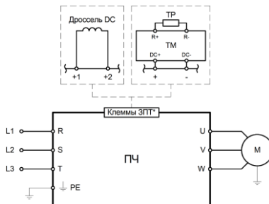
Рис. 3.2.7 — Подключение силовых клемм для моделей LCI-GY/PY-6
