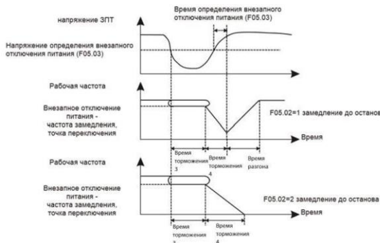
Рис. 6.9 — Действия при внезапном отключении питания
