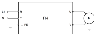
Рис. 3.2.1 — Подключение силовых клемм для моделей LCI-GY/PY-1
